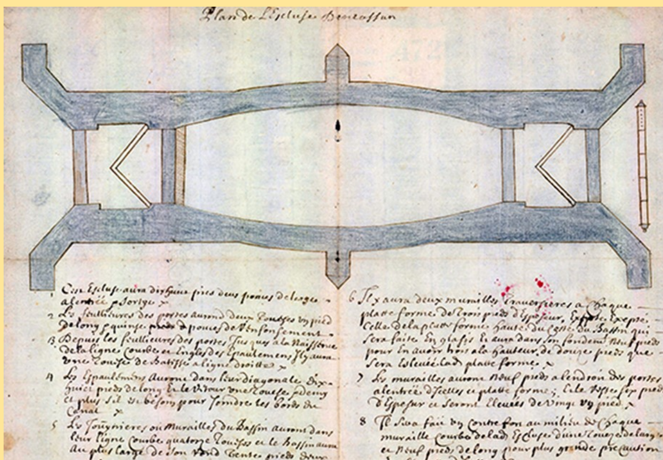
Plan de l'écluse d'En Cassan 1671. Archive VNF.
